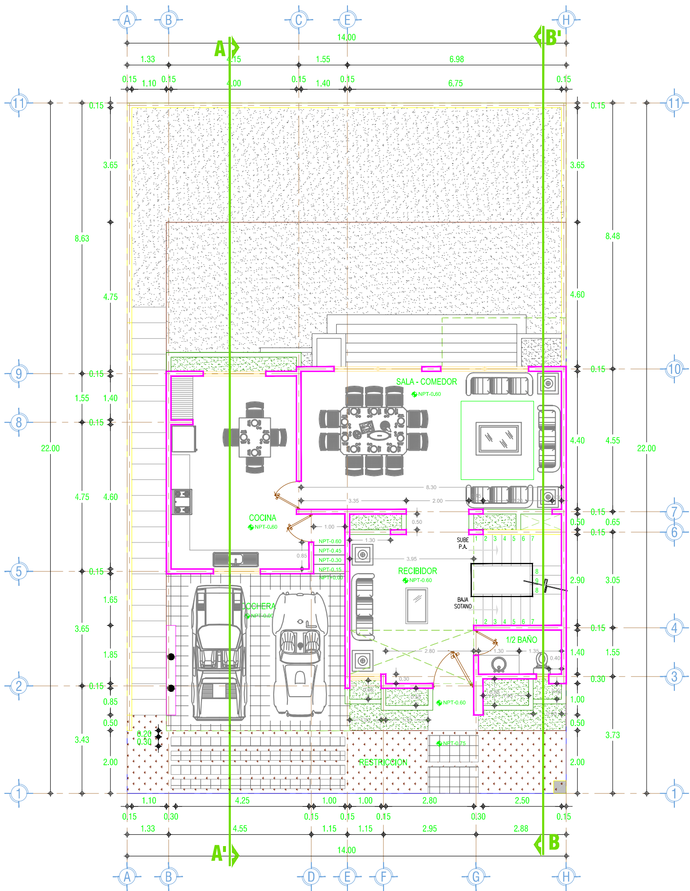
PLANTA BAJA ARQUITECTONICA Escala 1:100
